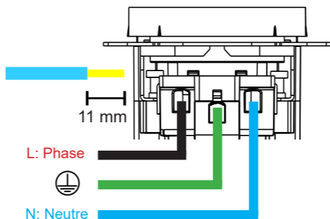
Schéma de câblage pour EK-PWS-FR-USB
