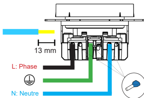
Schéma de câblage pour EK-PWS-FR
