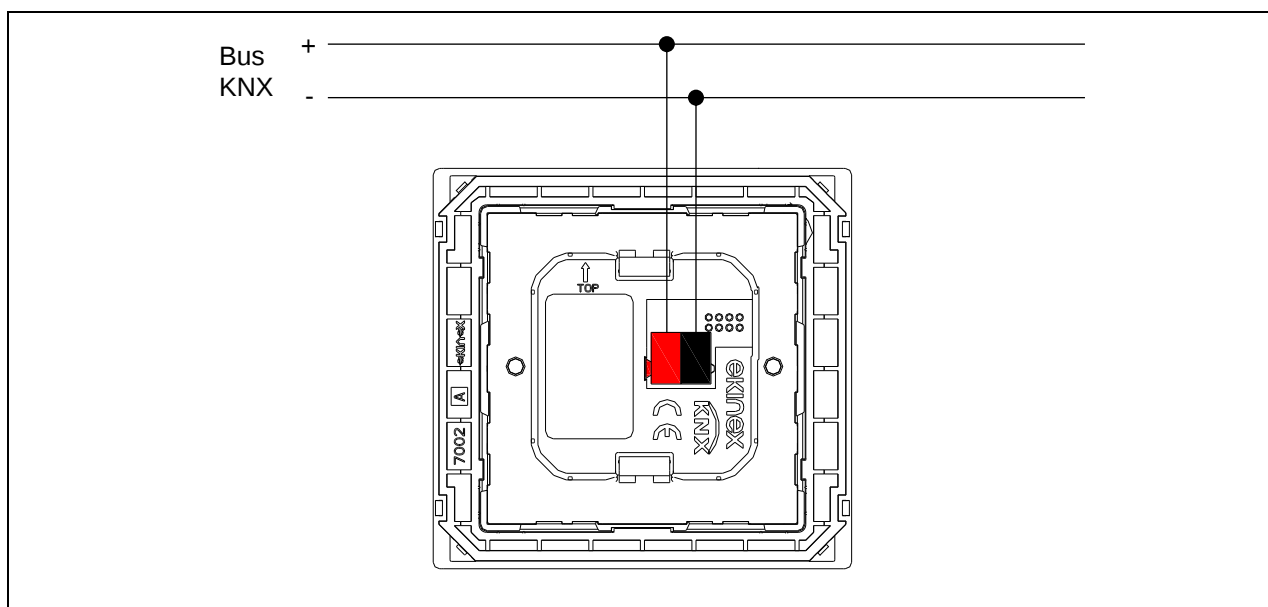
Collegamento dell'apparecchio alla linea bus
