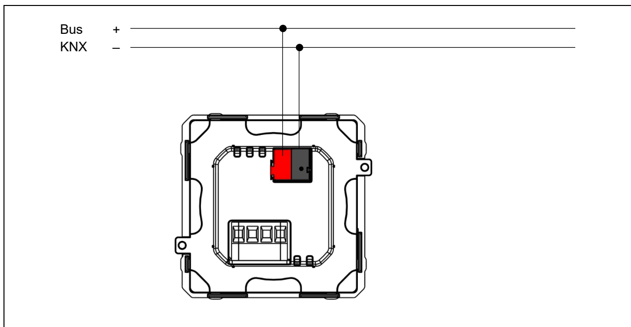
Figura 2 - Collegamento dell'apparecchio alla linea bus
